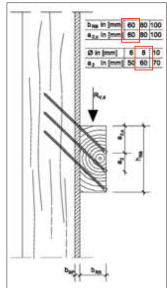
Mindestbreite des Pfostens b_{1,min} = 60 \text{ mm}
