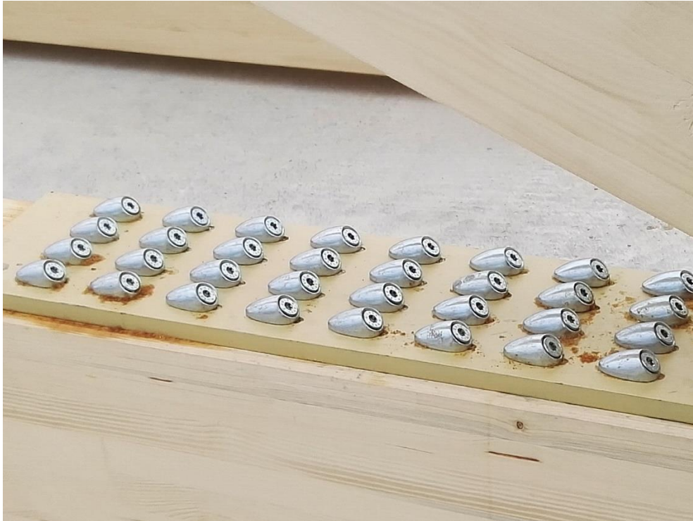
Bild 4: Zuganschluss der Stahlplatte an den Untergurt mit ASSY® plus VG Schrauben in Kombination mit Winkelscheiben 45°
