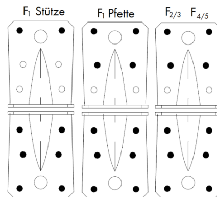
Winkelverbinder Typ A 55x70x70x2,5mm Art. Nr. 5390 201 070
