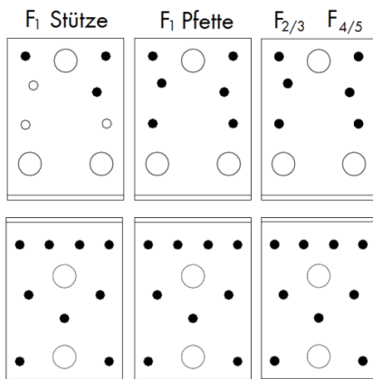
Winkelverbinder Typ A 65x90x90x2,5mm Art. Nr. 5390 200 090
