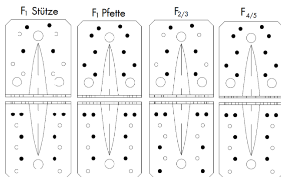
Winkelverbinder Typ A 90x105x105x3,0mm Art. Nr. 5390 201 105
