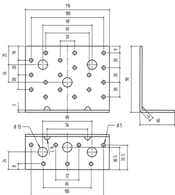
Winkelverbinder Typ HS 48x90x116x3mm Art. Nr. 0681 048 116
