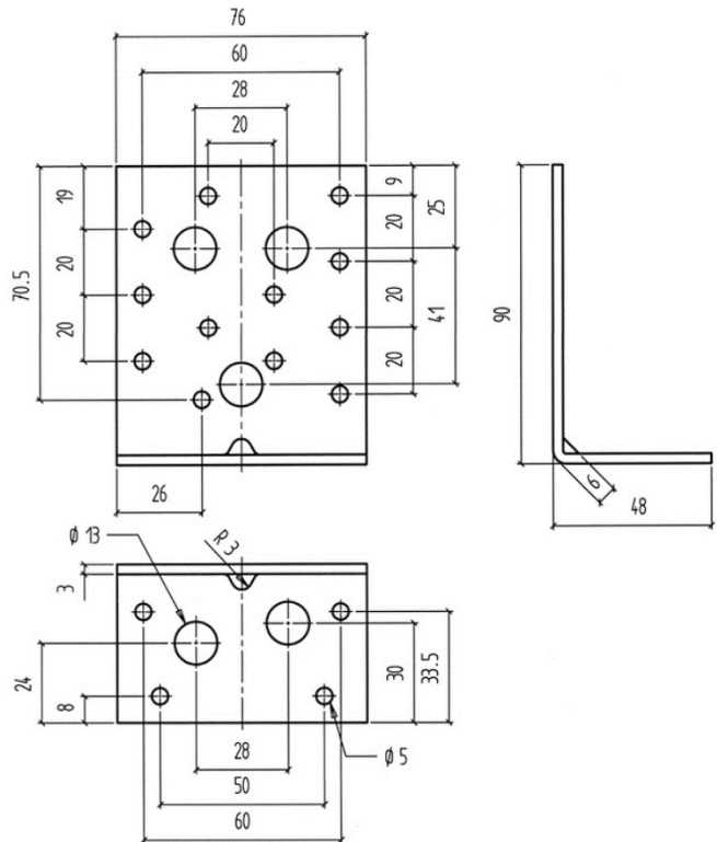
Winkelverbinder Typ HS 48x90x76x3mm Art. Nr. 0681 048 76
